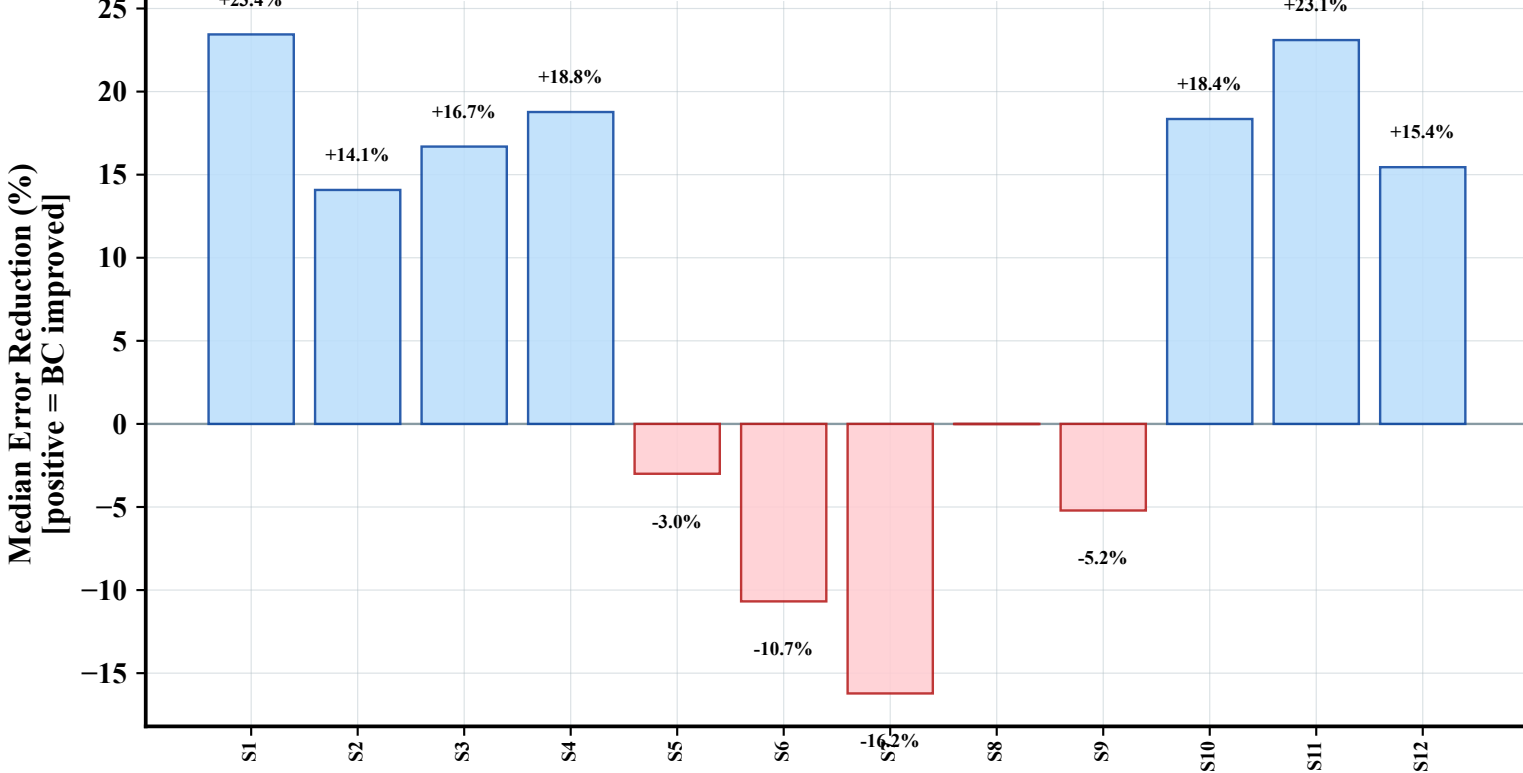
(d) Median Absolute Error Reduction After QDM
